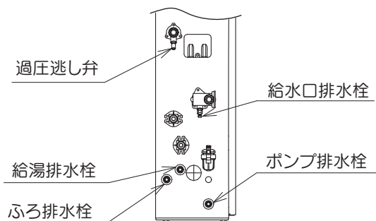
排水栓位置図
