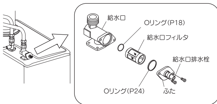
(FP) (FFP) (FFK) タイプ
